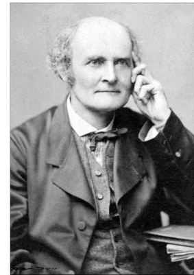
Arthur Cayley
